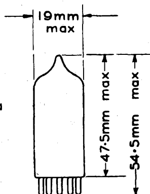
B7G Base
