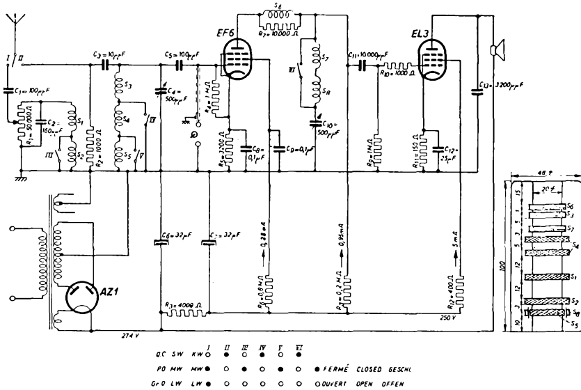
SCHALTUNGSBEISPIEL OHNE PATENTBLIGO UNSERERSEITS EXEMPLE D'UN SCHEMA DE MONTAGE DONNE SANS GARANTIE EN REGARD DE DROITS DE BREVETS D'INVENTION SPECIMEN OF CIRCUIT DIAGRAM WITHOUT ANY GUARANTEE AS TO PATENTRIGHTS 23244 Circuit diagram.
