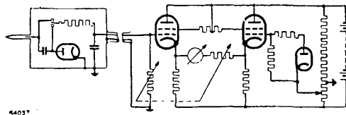
Skeleton circuit.
