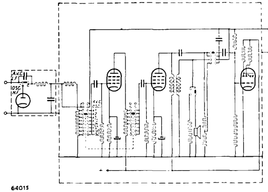
Skeleton circuit.
